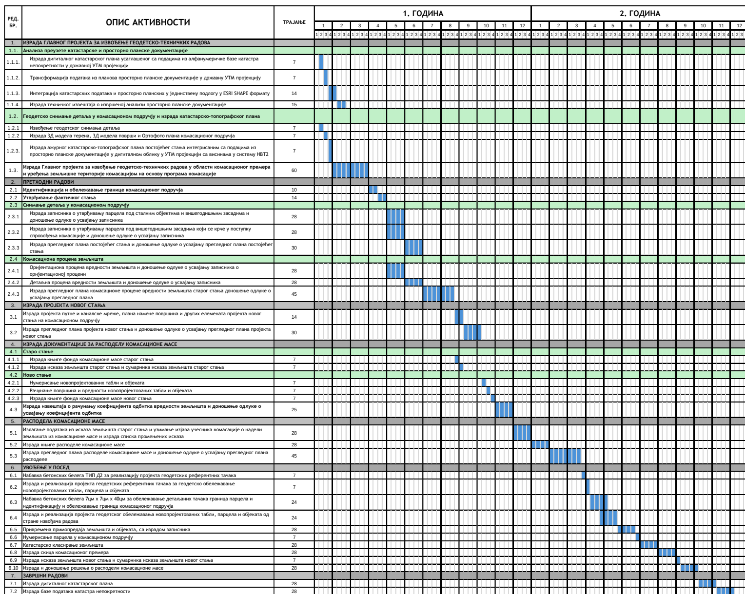
Дијаграм 3: Дијаграм активности на реализацији геодетско-техничких радова
