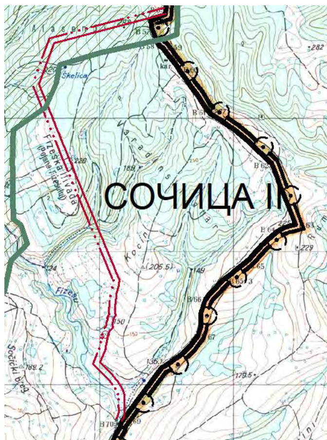
Слика 9: Могући распоред пољозаштитних шумских појасева на КО Сочица II
