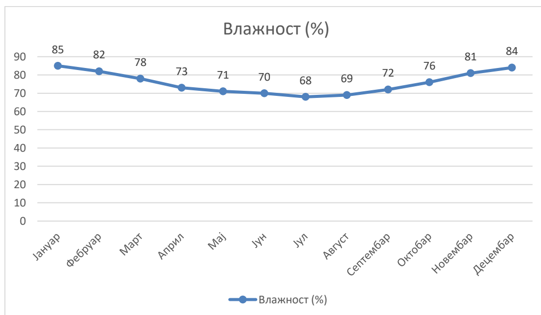
Графикон 3: Просечна релативна влажност ваздуха по месецима (%)
